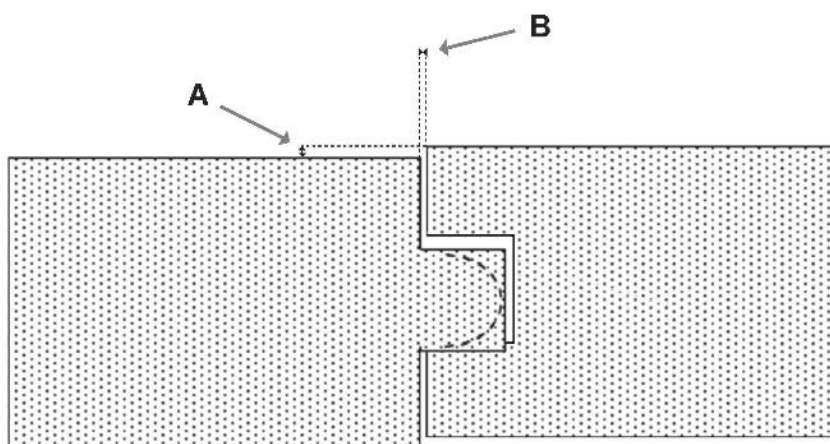
Figuur 2 - Bepaling afmetingen hoogteverschil en kier bij mes en groef
