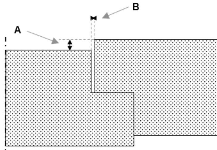
Figuur 1 - Bepaling afmetingen hoogteverschil en kier bij standaard sponning
